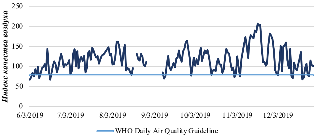
Выбросы твердых частиц PM 2.5 в Ташкенте, июнь-декабрь 2019 г.
