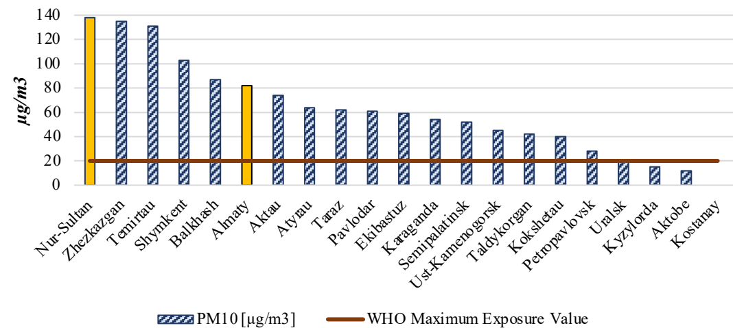
Среднегодовая концентрация PM10, 2015-2017
